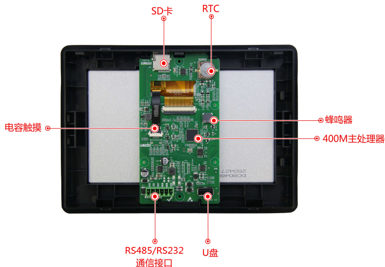
图 1-2 硬件配置图
