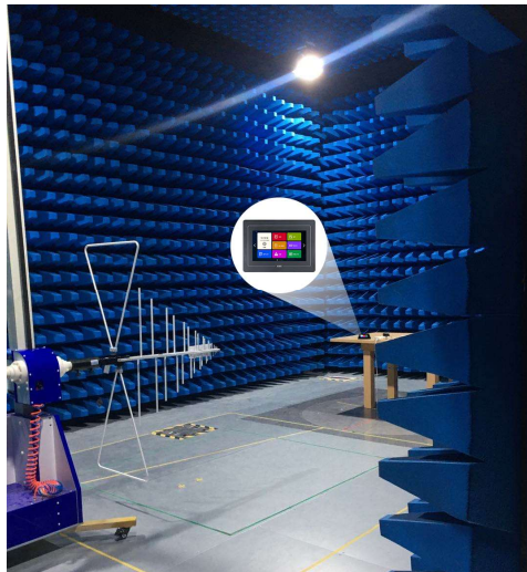
图 5-4 RE 测试图
